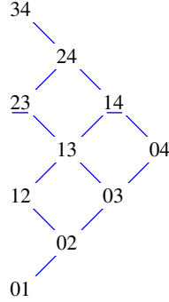
Fig. 2. \mathbb{Y}_{2,5}
